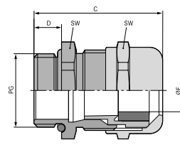
SKINTOP® MSR
